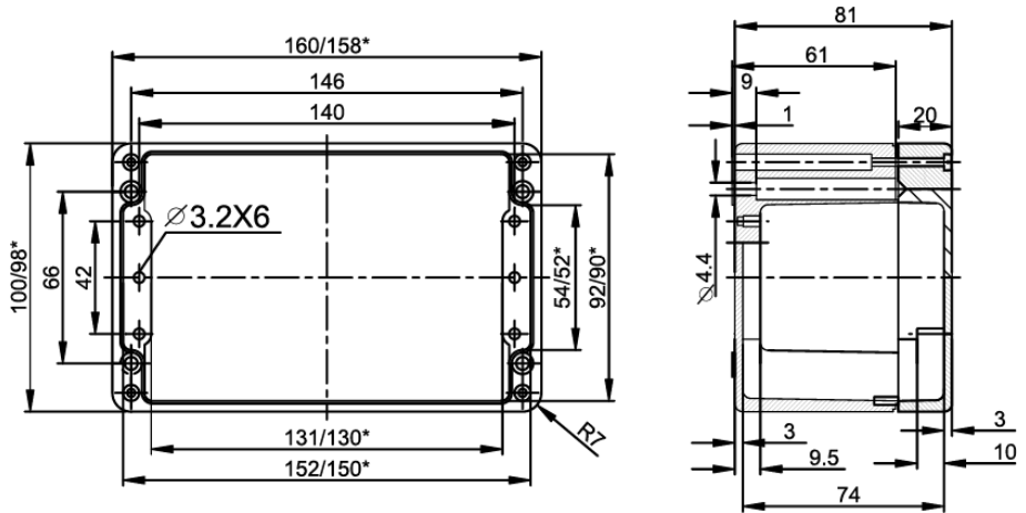
Рисунок 1. Габаритные и крепежные размеры блока.
