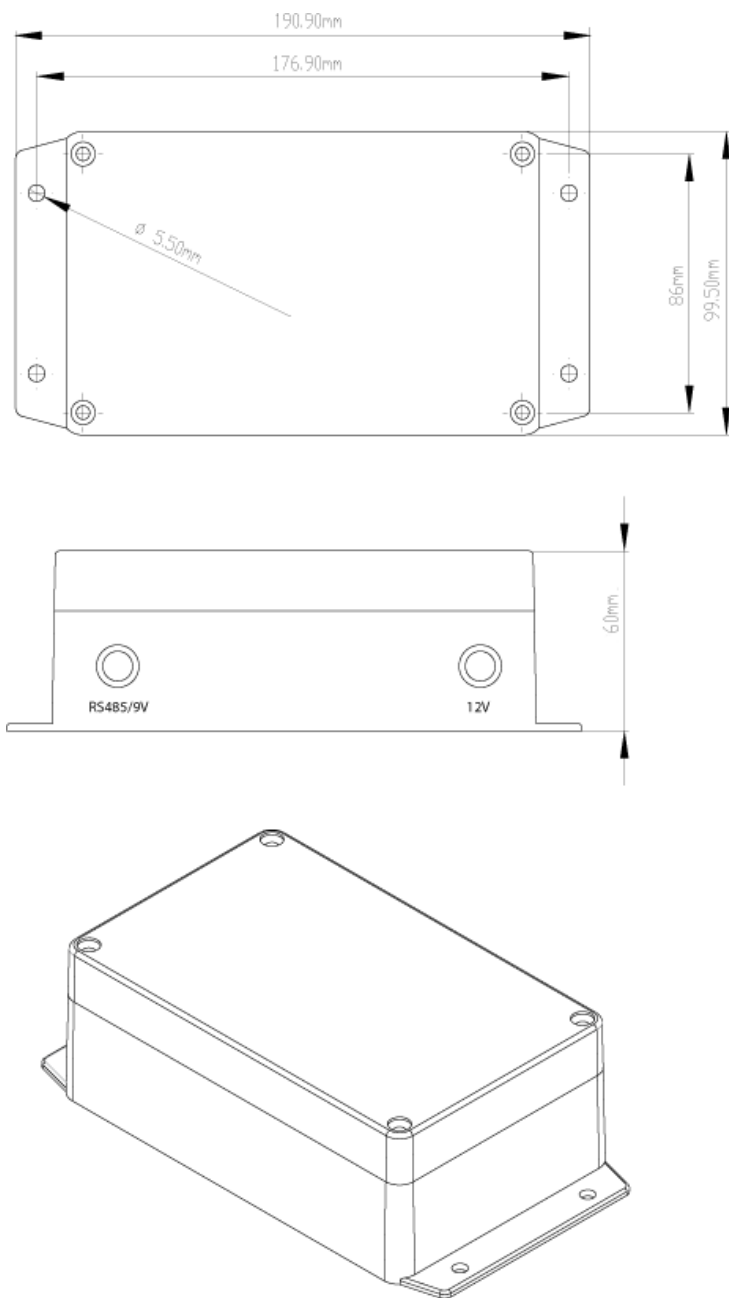
Рисунок 1. Внешний вид, габаритные и крепежные размеры блока.
